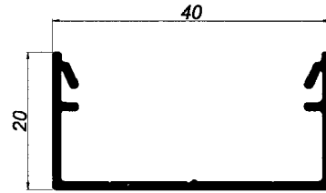
02003 U DE PASAMANOS DE 40
