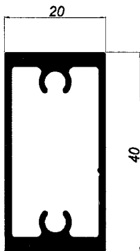
02024 PILAR DE 40X20
