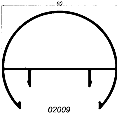
02009 PASAMANOS REDONDO DE 60 CLIP
