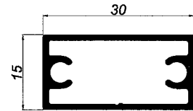
02006 RECTANGULO AUTORROSCANTE DE 30x15
