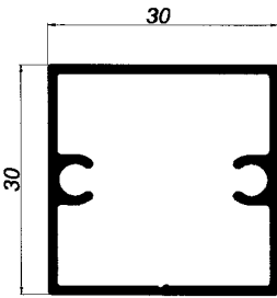
02007 CUADRADO AUTORROSCANTE DE 30x30
