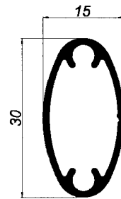
02005 OVALO DE 30x15
