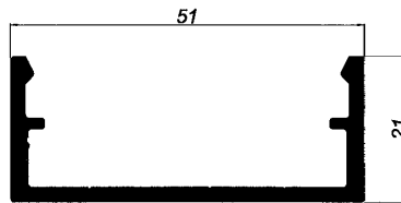
02023 U DE PASAMANOS DE 51
