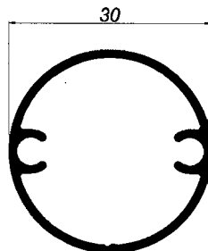
02008 REDONDO AUTORROSCANTE DE 30
